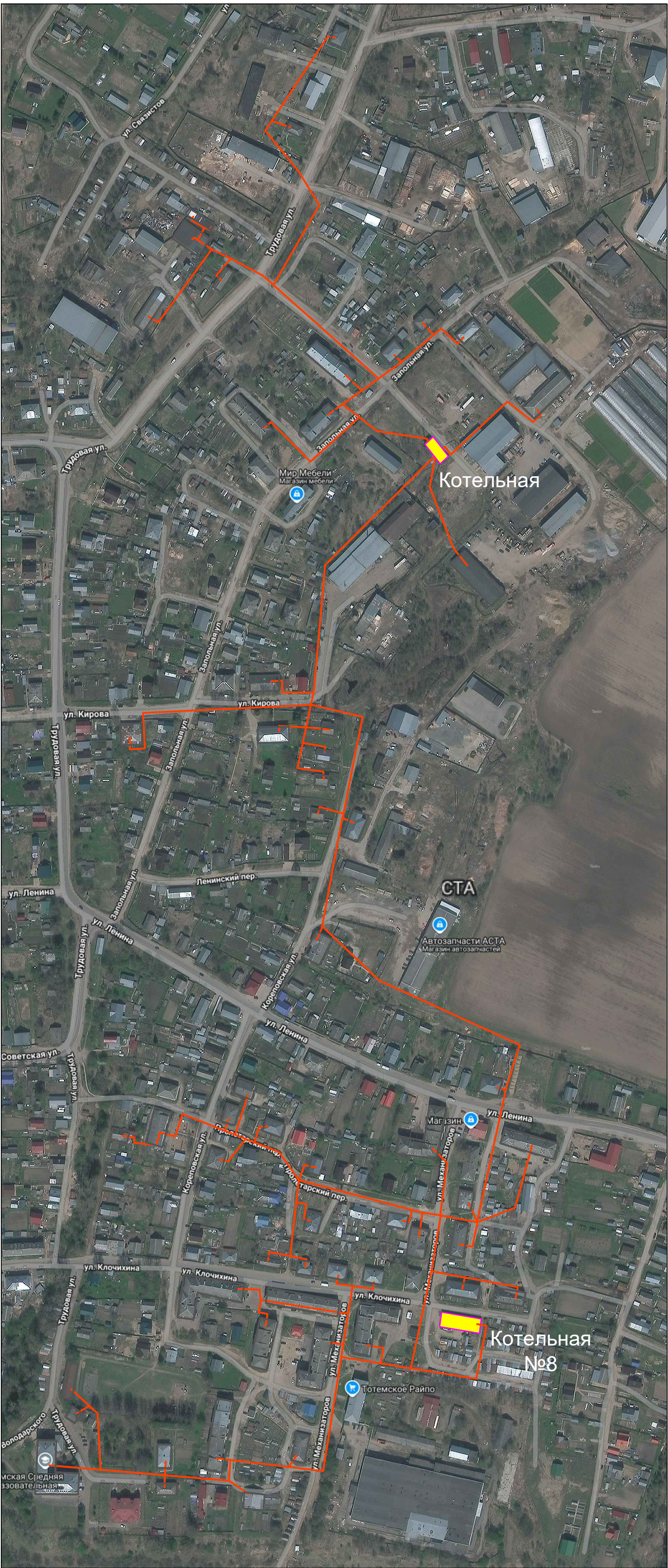
Схема тепловой сети от котельной №8, г. Тотьма
