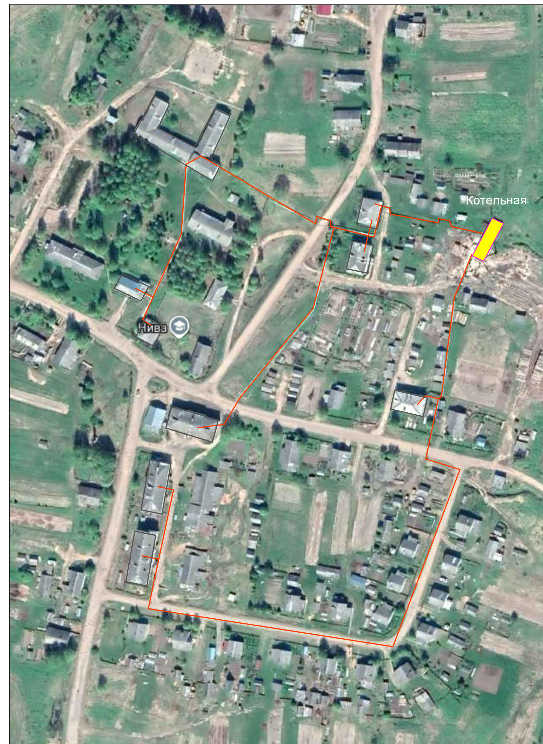
Схема теплоснабжения д. Мосеево, фрагмент территории
